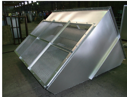
建築設備用外気取入口
