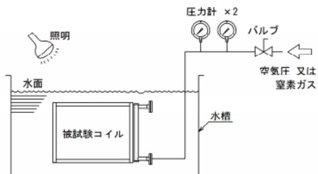
熱交換器気密試験設備並試験要領
