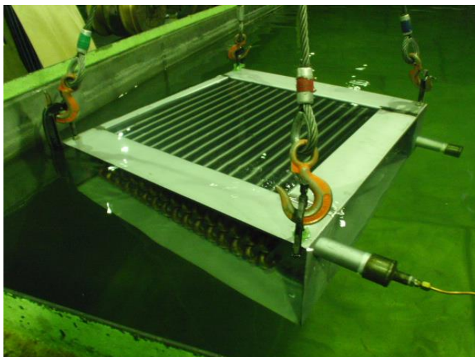
熱交換器気密試験設備並試験要領
